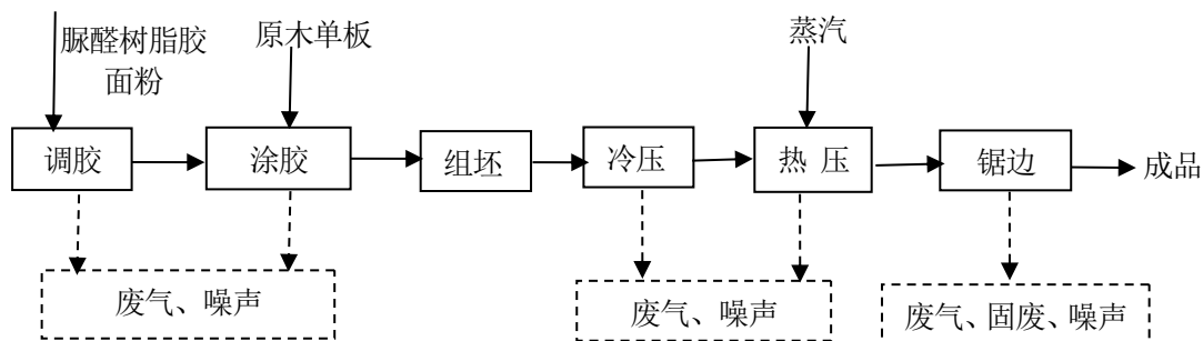
图2 本项目工艺流程及产污环节示意图
